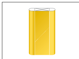
MP2 - 1x3, varenr. 82221, 1268 (b) x 2225 (h) x 320 (d) mm
