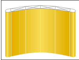
MP1 - 4x3, varenr. 82204 2875 (b) x 2255 (h) x 840 (d) mm MP2 - 4x3, varenr. 82214 3150 (b) x 2225 (h) x 960 (d) mm
